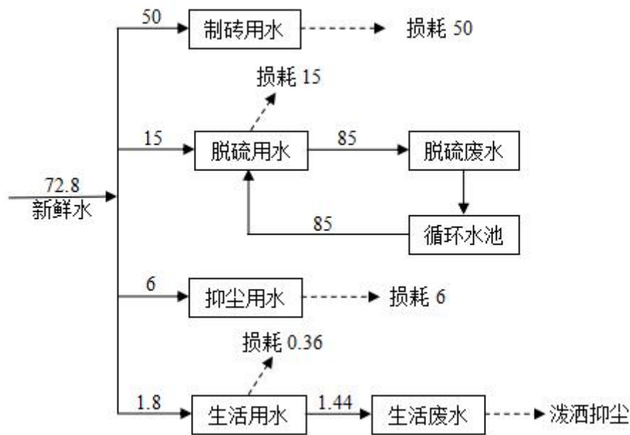
图 4-2 项目水平衡图 单位：m 3 /a
