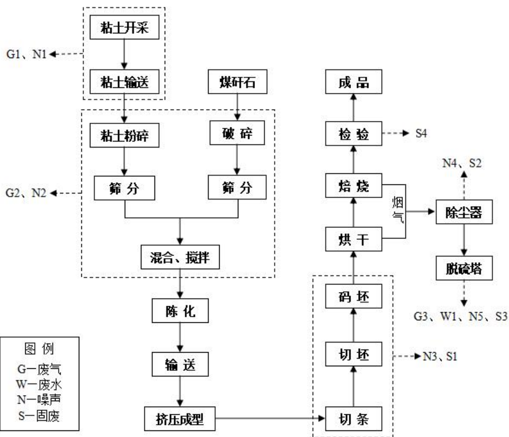
图 4-3 项目生产工艺流程及产污环节图
