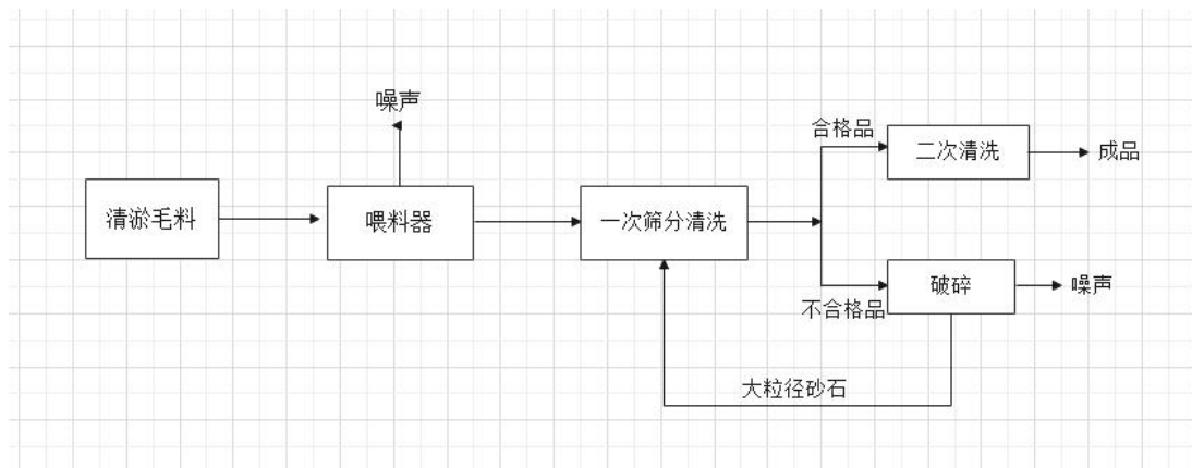
图2-4 运营期生产工艺流程及产物环节示意图
