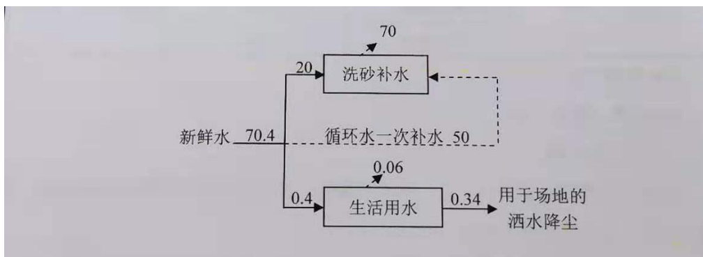
图 2-3 项目水平衡图(m 3 /d)
